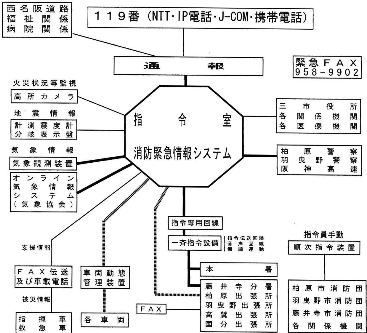
資料2 - 8 消防通信指令系統図
