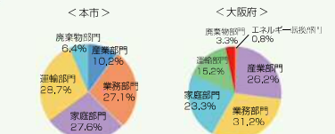
▲本市(左)と大阪府(右)の温室効果ガス排出量部門別割合(2021年度)
