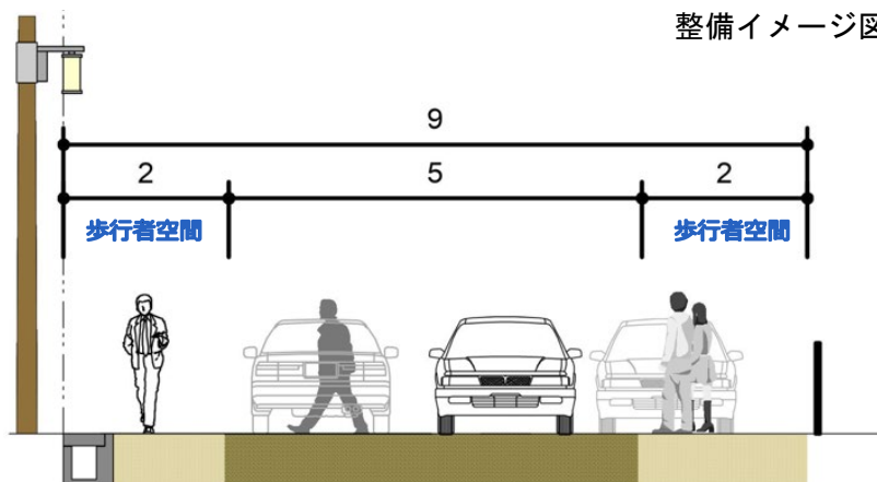
標準断面
