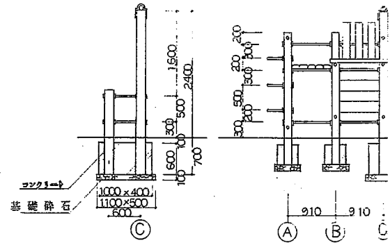
① 通り 軸組図
